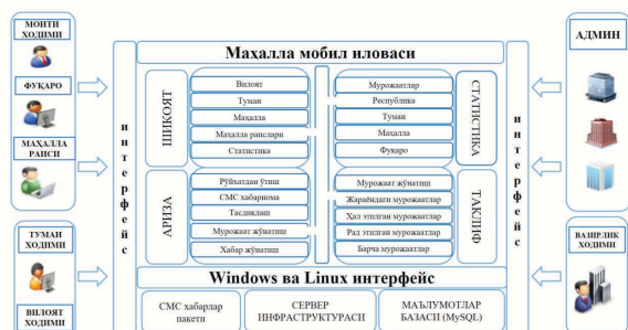
1-расм. Маҳалла ахборот тизими умумий структураси
